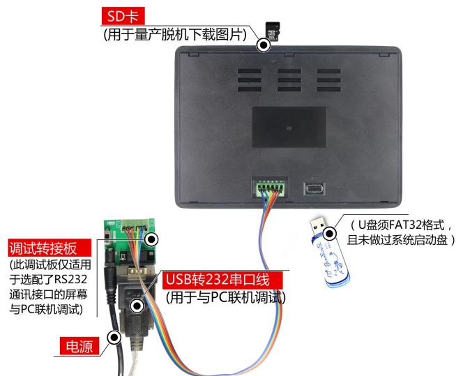
图 1-3 RS232 调试图
