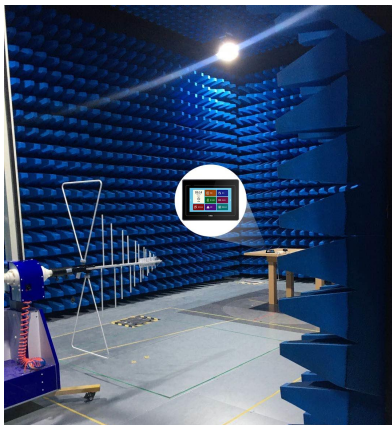
图 6-5 辐射测试图
