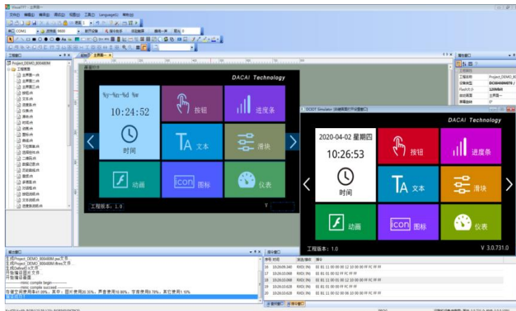
图 12-1 VisualTFT 主界面
