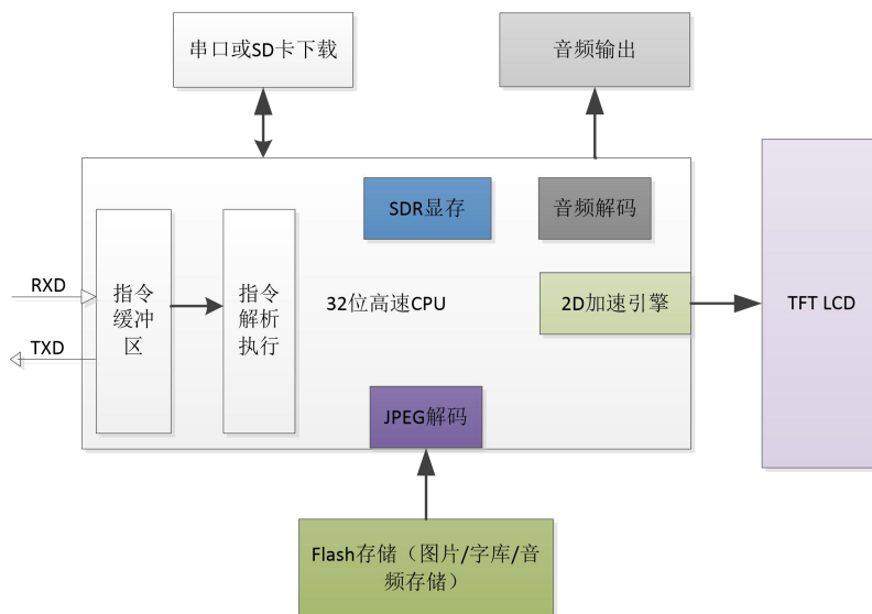
图 11-1 M 系列串口屏内部结构图
