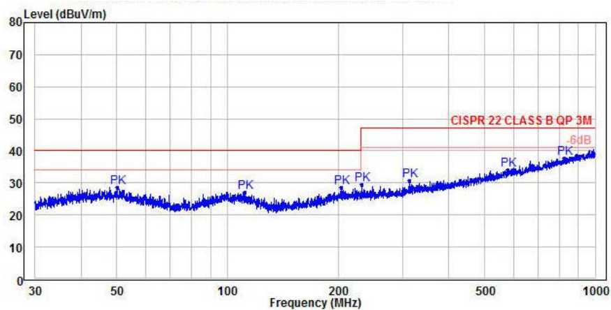
图 6-6 辐射测试水平方向
