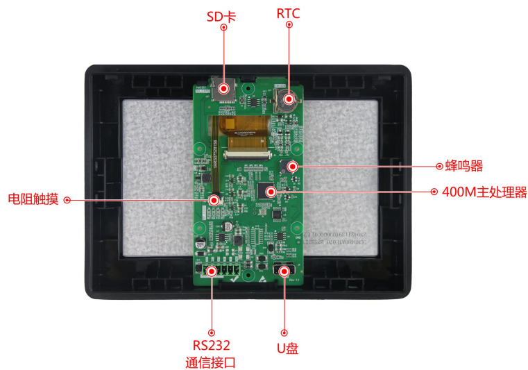
图 1-2 硬件配置图
